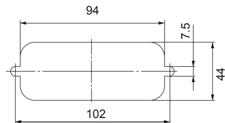
切割尺寸圖 Panel cutout dimension
