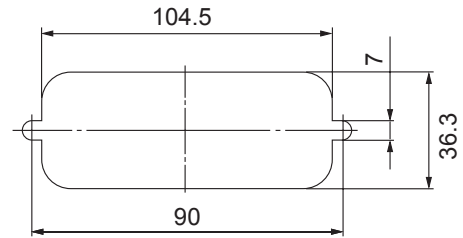
切割尺寸圖 Panel cutout dimension
