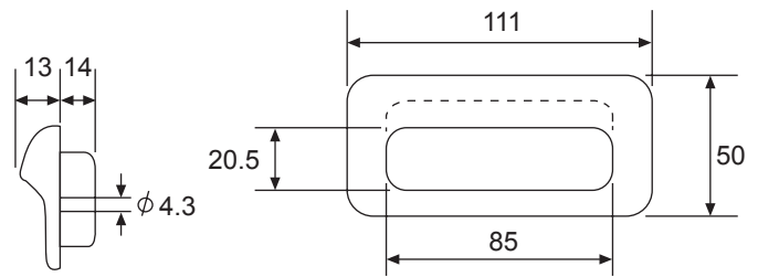
切割尺寸圖 Panel cutout dimension
